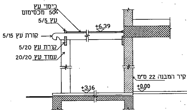
פרט פרגולה
